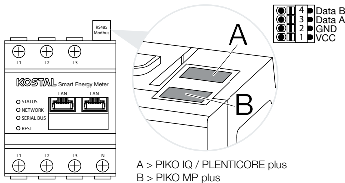
Abb. 8: RS485 Schnittstellen
